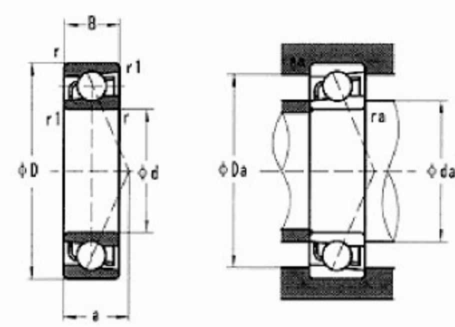
角接触轴承尺寸表 size of angular contact ball bearing
